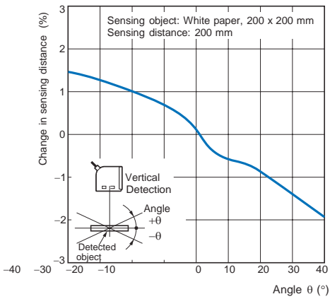
E3S-CL2 Vertical
